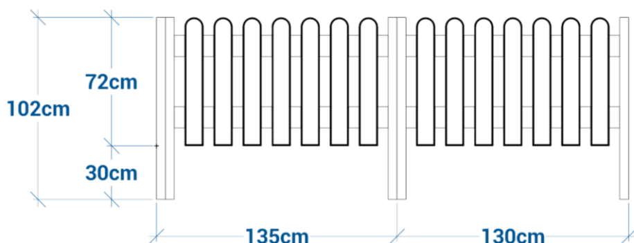
Module intermédiaire + un poteau début/fin
