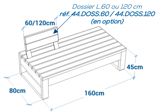
Banquette - réf. 65.1
