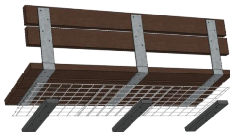
Assises fixées sur des ferrures acier galvanisé Fixation au gabion à l'aide de planches 8,2x3 cm
