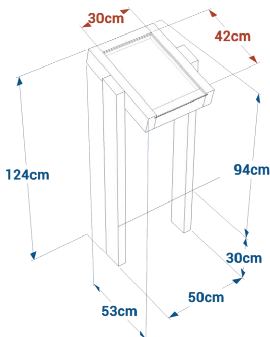
Poteaux rallongés pour scellement
