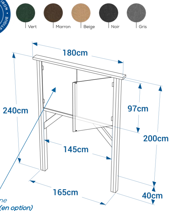
Poteaux rallongés pour scellement
