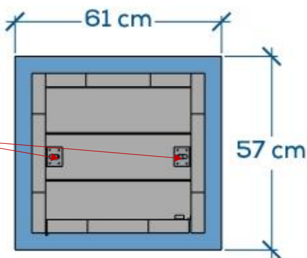
Profondeur de dalle 15 cm
