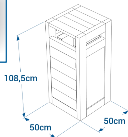
Porte-sac 130 L
